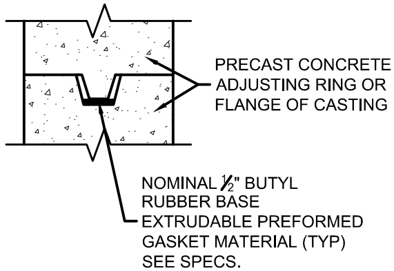
GASKET
